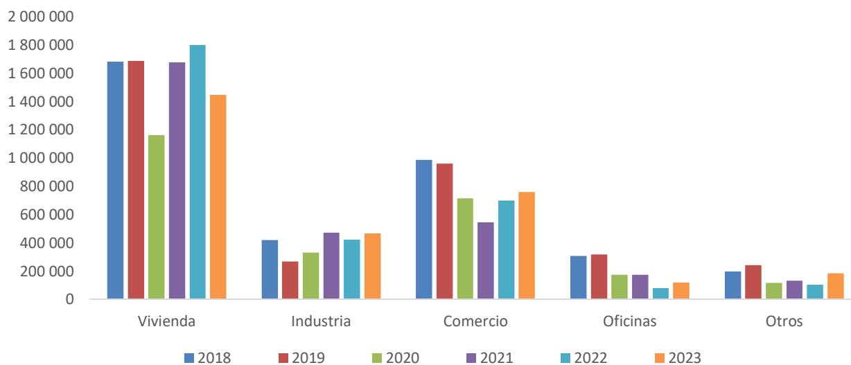
Gráfico 14. Área de construcción tramitada por tipo de edificio. Al primer semestre de cada año
